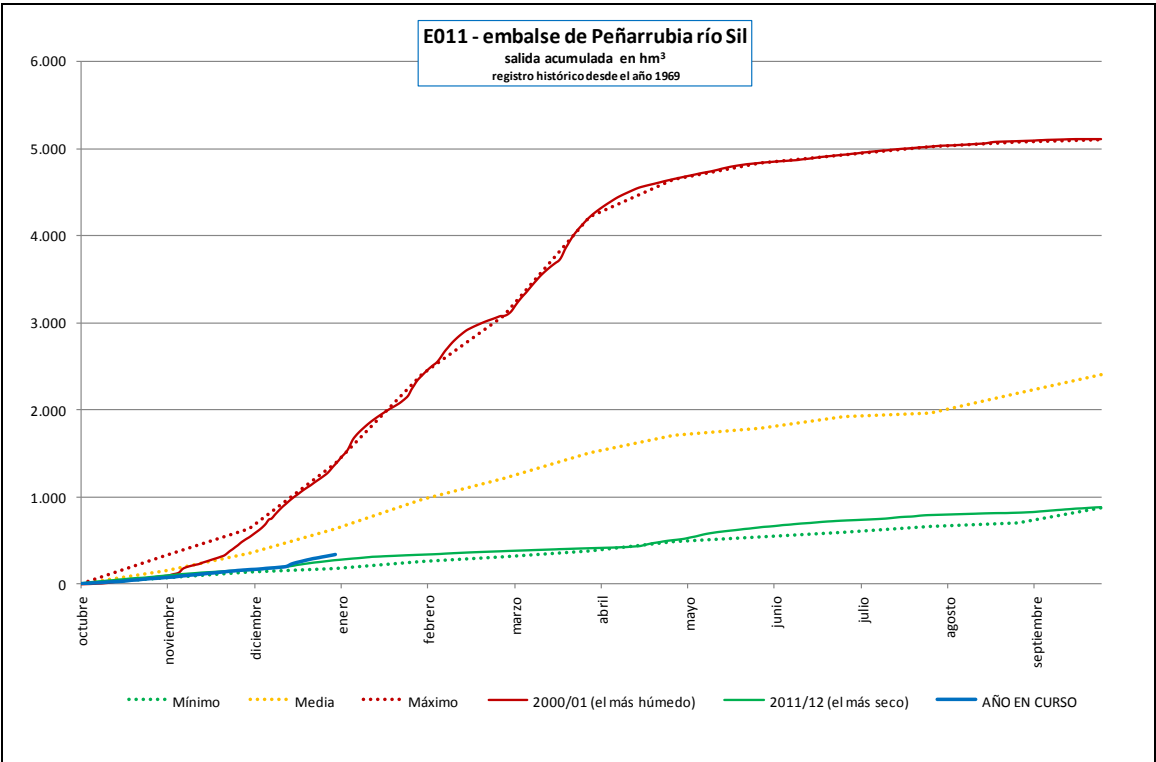
Embalse de Peñarrubia (Caudales de salida al río) (Datos consolidados diarios disponibles hasta el 31 de diciembre de 2012)
