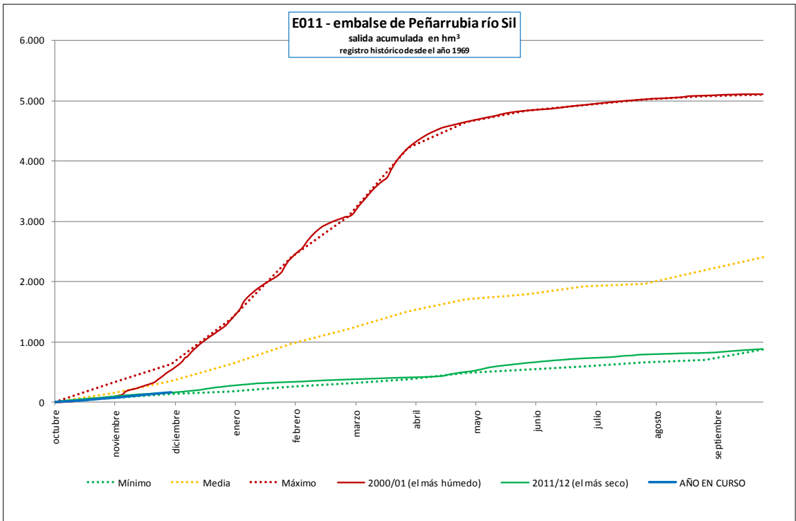
Embalse de Peñarrubia (Caudales de salida al río) (Datos consolidados diarios disponibles hasta el 30 de noviembre de 2012)
