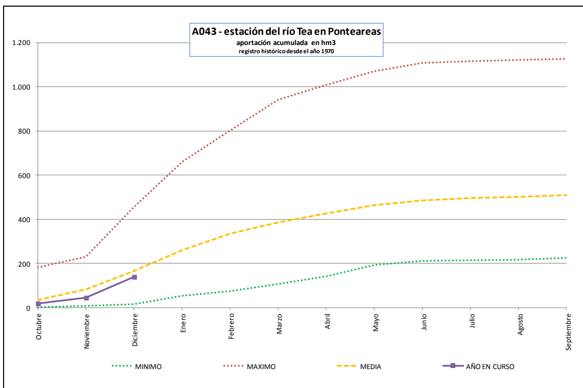
Estación de aforo A043 del río Tea en Pontearreas
