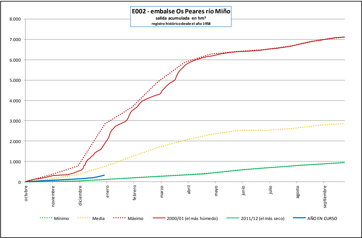
Embalse de Os Peares (Caudales de salida al río)
