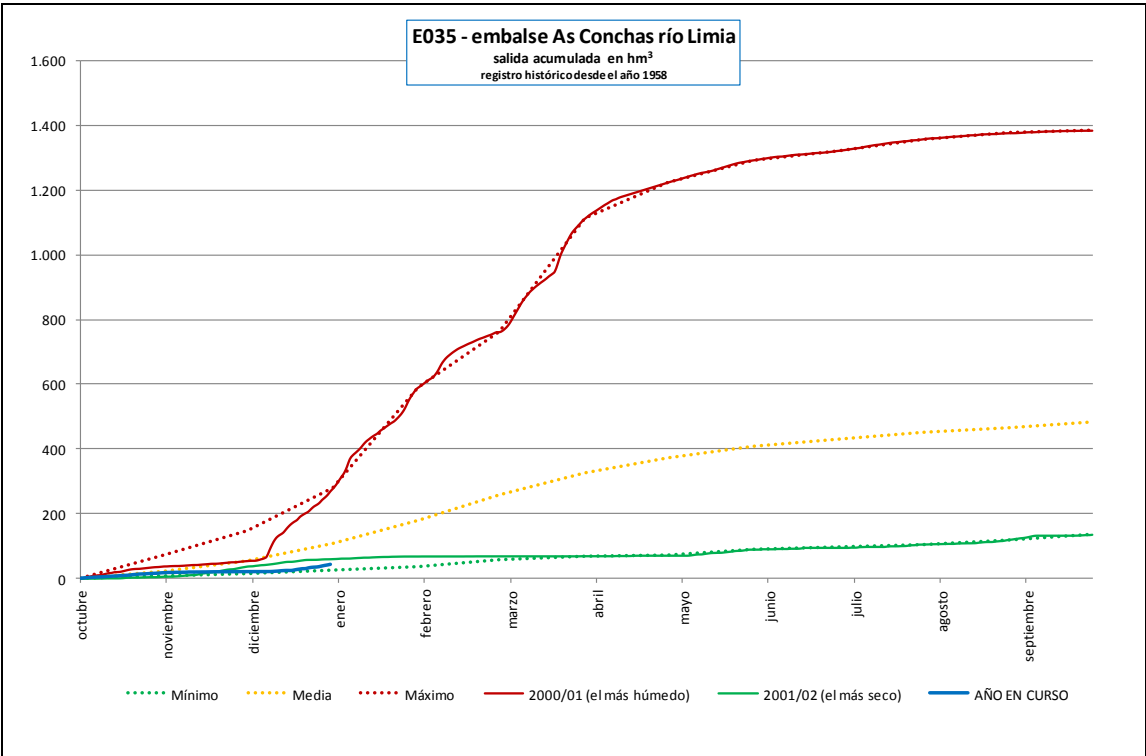
Embalse de As Conchas (Caudales de salida al río)
