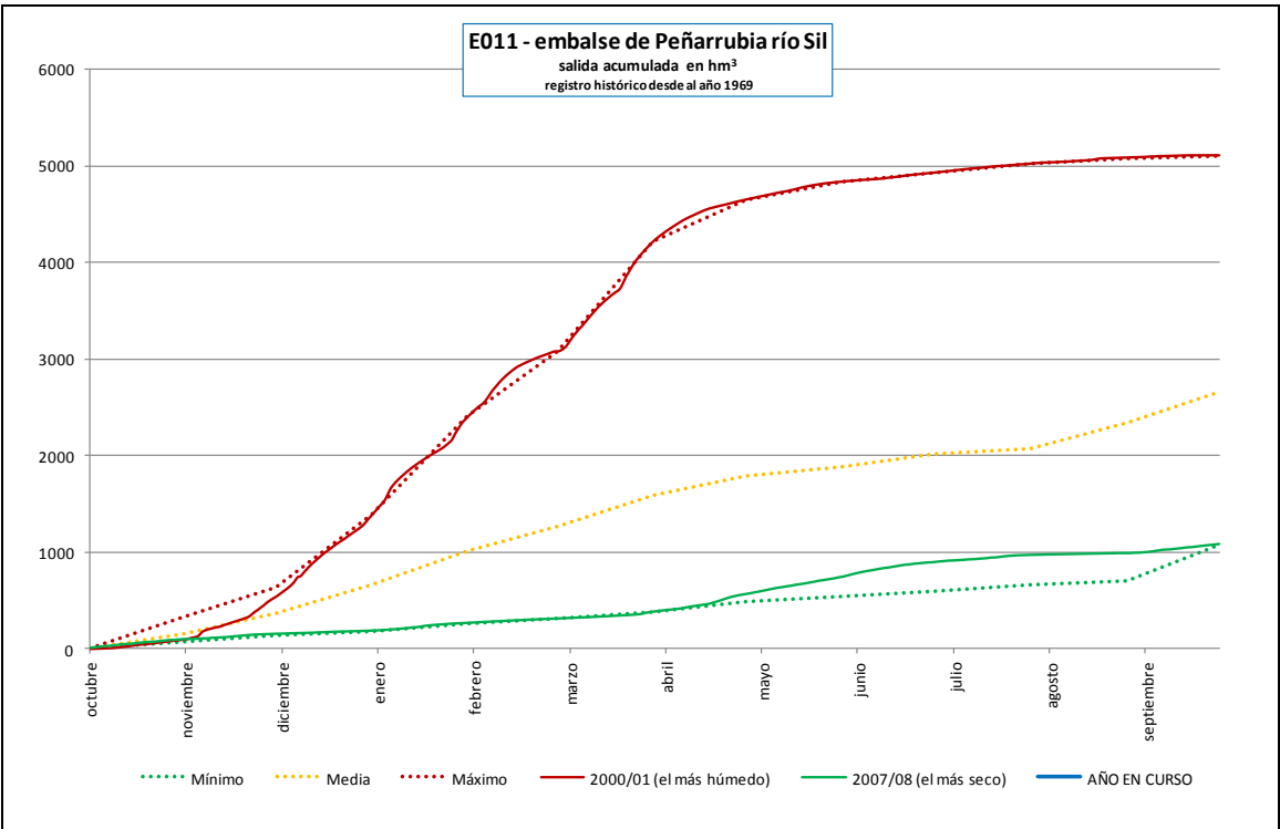
Embalse de Peñarrubia (Caudales de salida al río) (Datos consolidados diarios disponibles hasta el 30 de septiembre de 2012)
