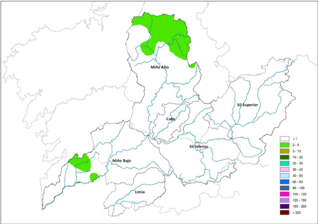
Precipitación media superficial en la última semana: 0,3 mm
