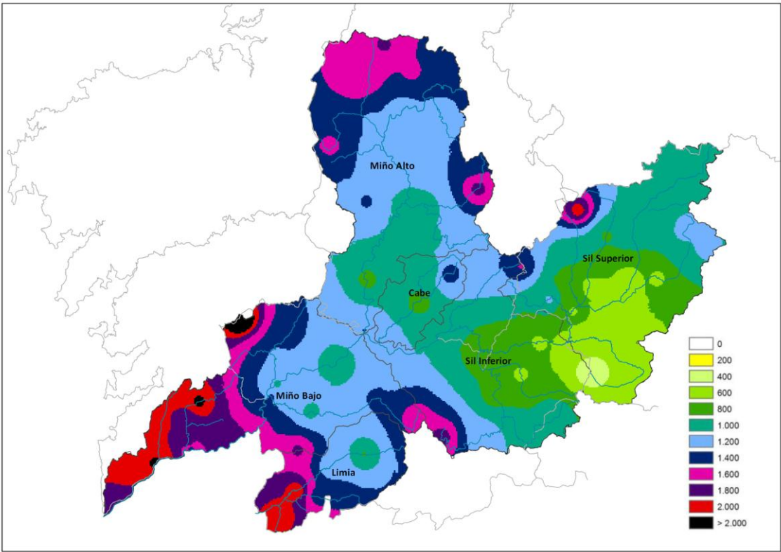
Precipitación media superficial desde el inicio del año hidrológico 1.091,0 mm
