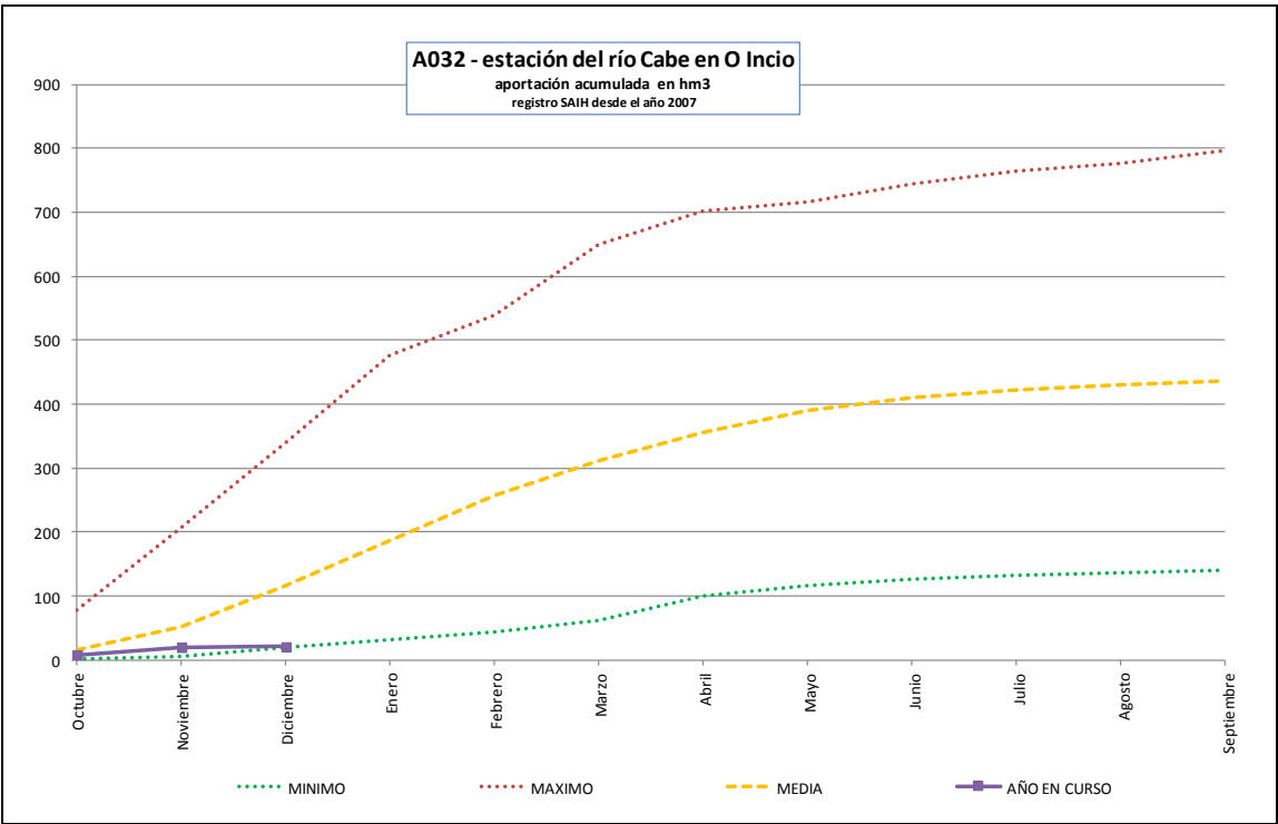
Estación de aforo A032 del río Cabe en O Incio
