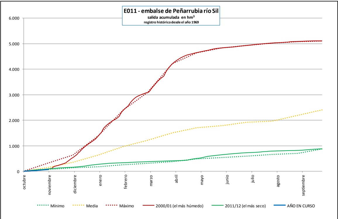
Embalse de Peñarrubia (Caudales de salida al río) (Datos consolidados diarios disponibles hasta el 31 de octubre de 2012)
