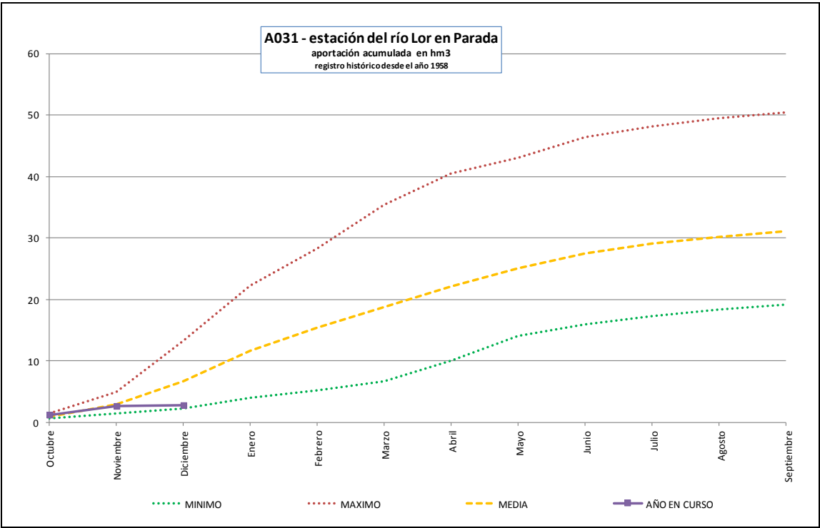
Estación de aforo A031 del río Lor en Parada (Los datos anteriores a 2008 corresponden a la estación de Iberdrola del Río Lor en A Ponte)
