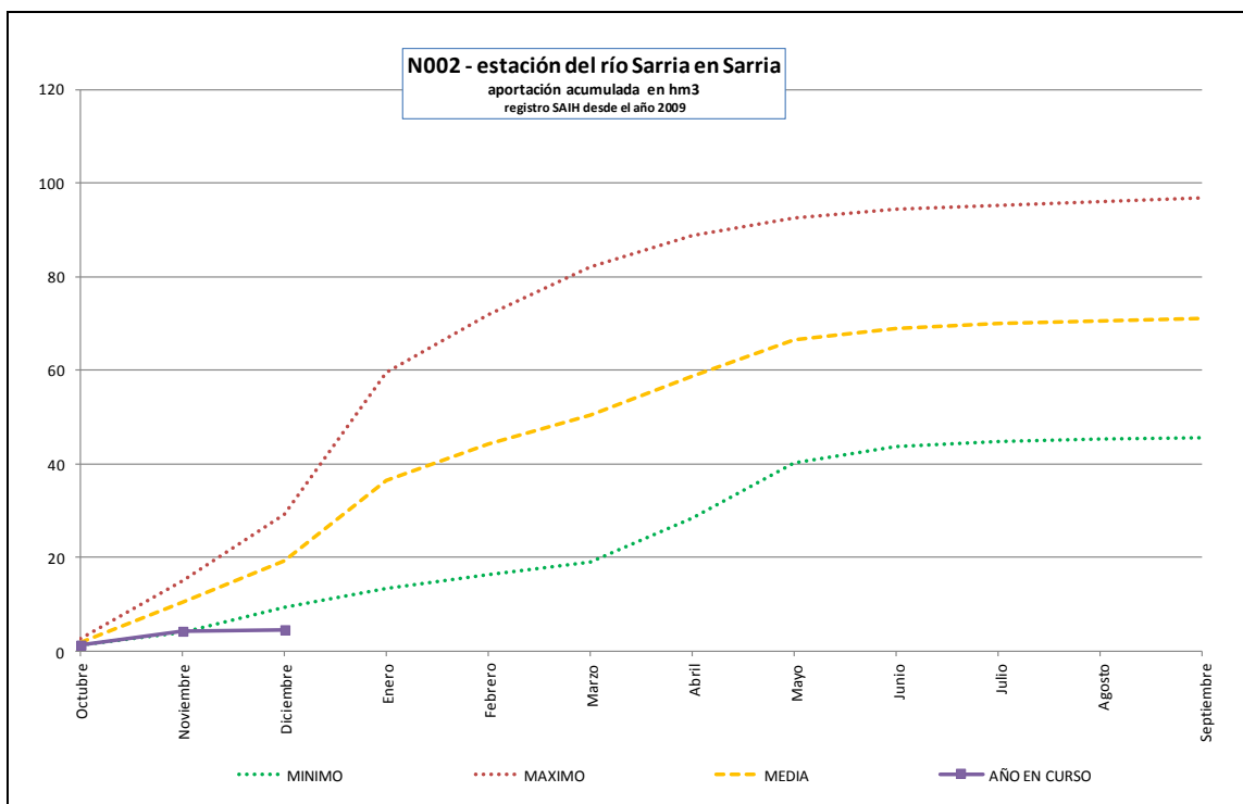
Estación de nivel N002 del río Sarria en Sarria (sólo se tiene completo el registro de los años hidrológicos 2010/11 y 2011/12)
