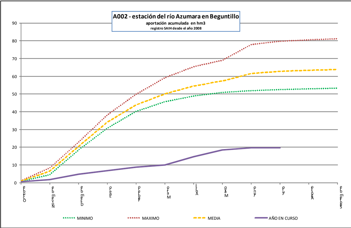
Estación de aforo A002 del río Azumara en Beguntillo
