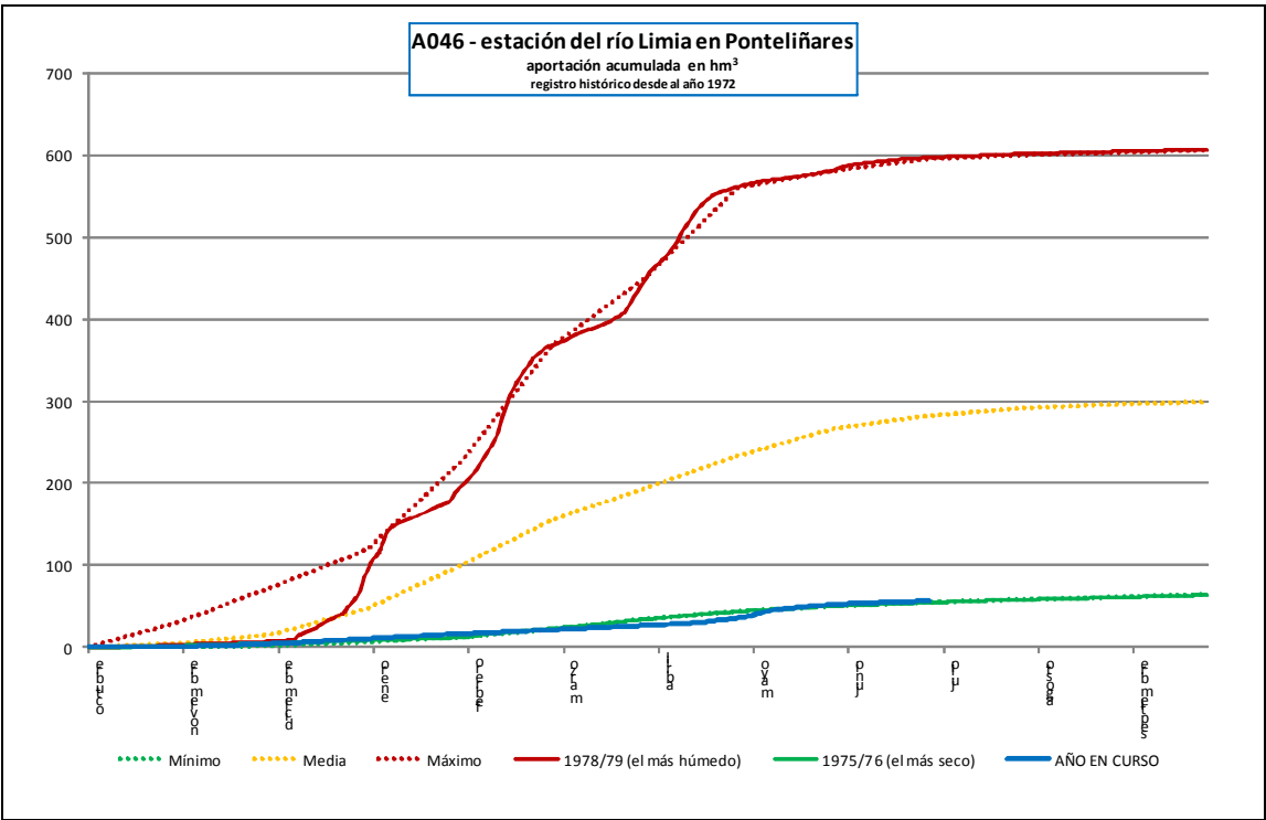
Estación de aforo A046 del río Limia en Ponteliñares
