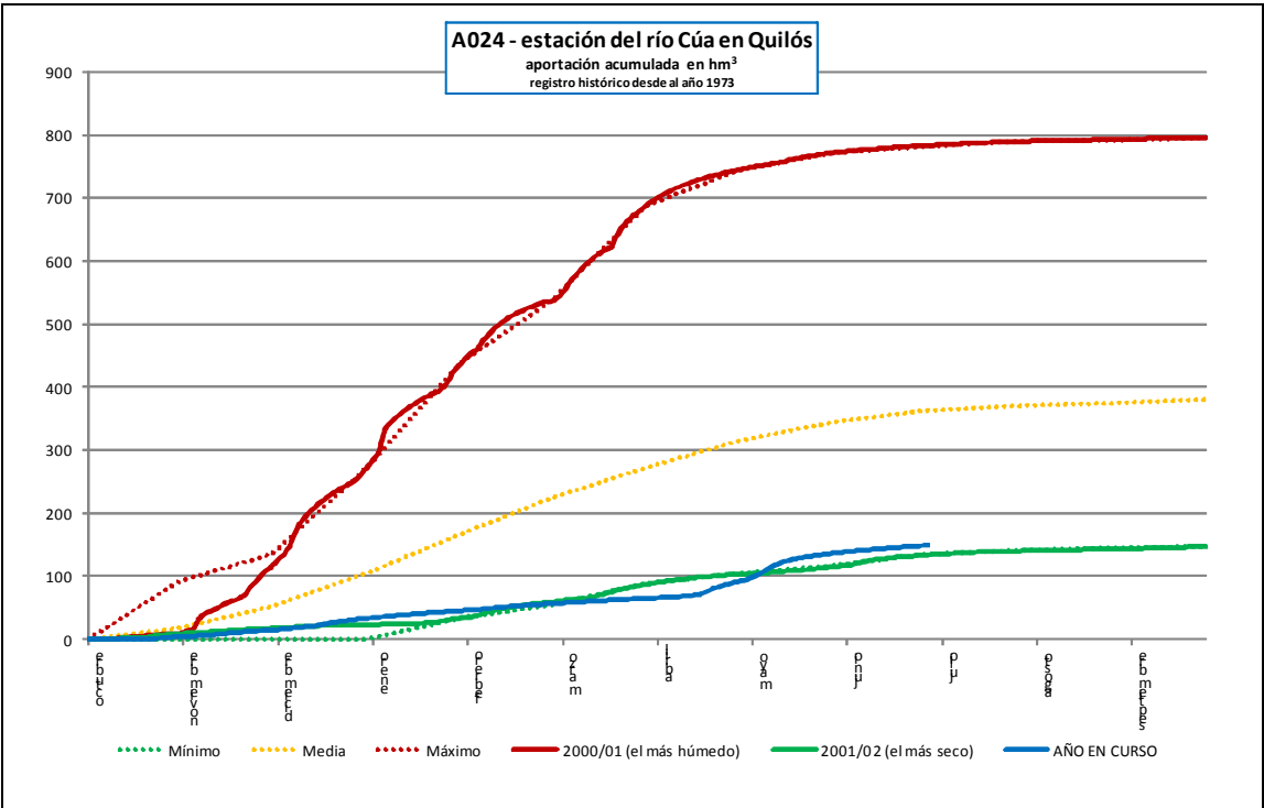
Estación de aforo A024 del río Cúa en Quilós
