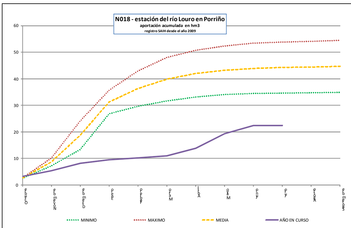
Estación de nivel N018 del río Louro en Porriño
