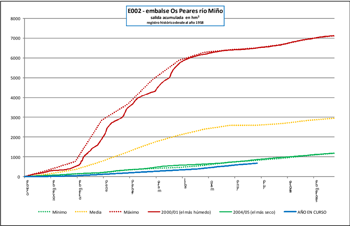
Embalse E002 del río Miño en Los Peares (Caudales de salida al río)
