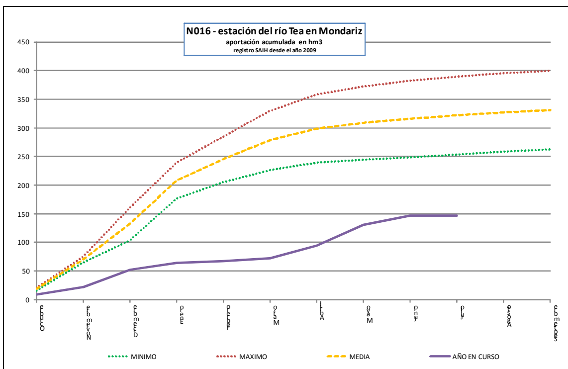
Estación de nivel N016 del río Tea en Mondariz
