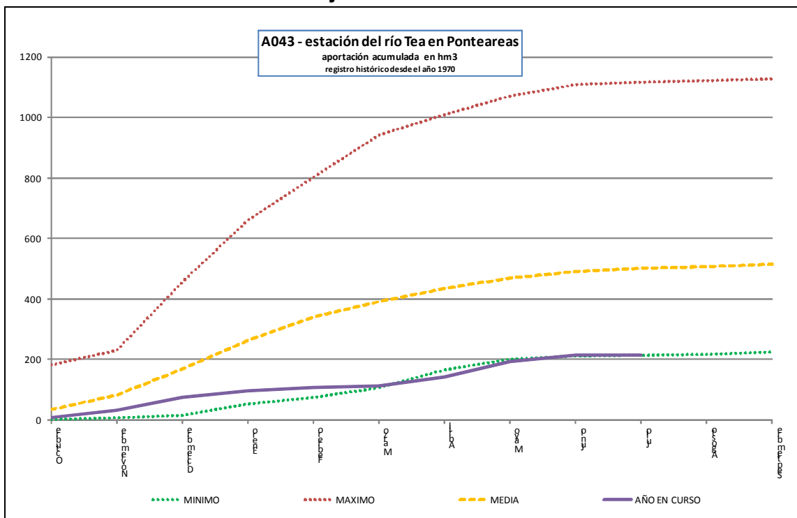
Estación de aforo A043 del río Tea en Ponteareas
