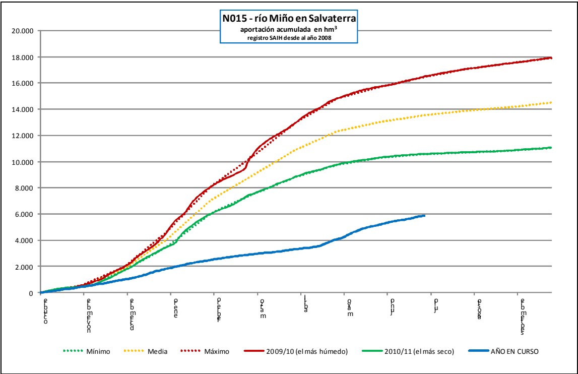
Estación de nivel N015 del río Miño en Salvaterra
