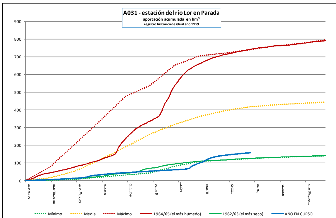
Estación de aforo A031 del río Lor en Parada
