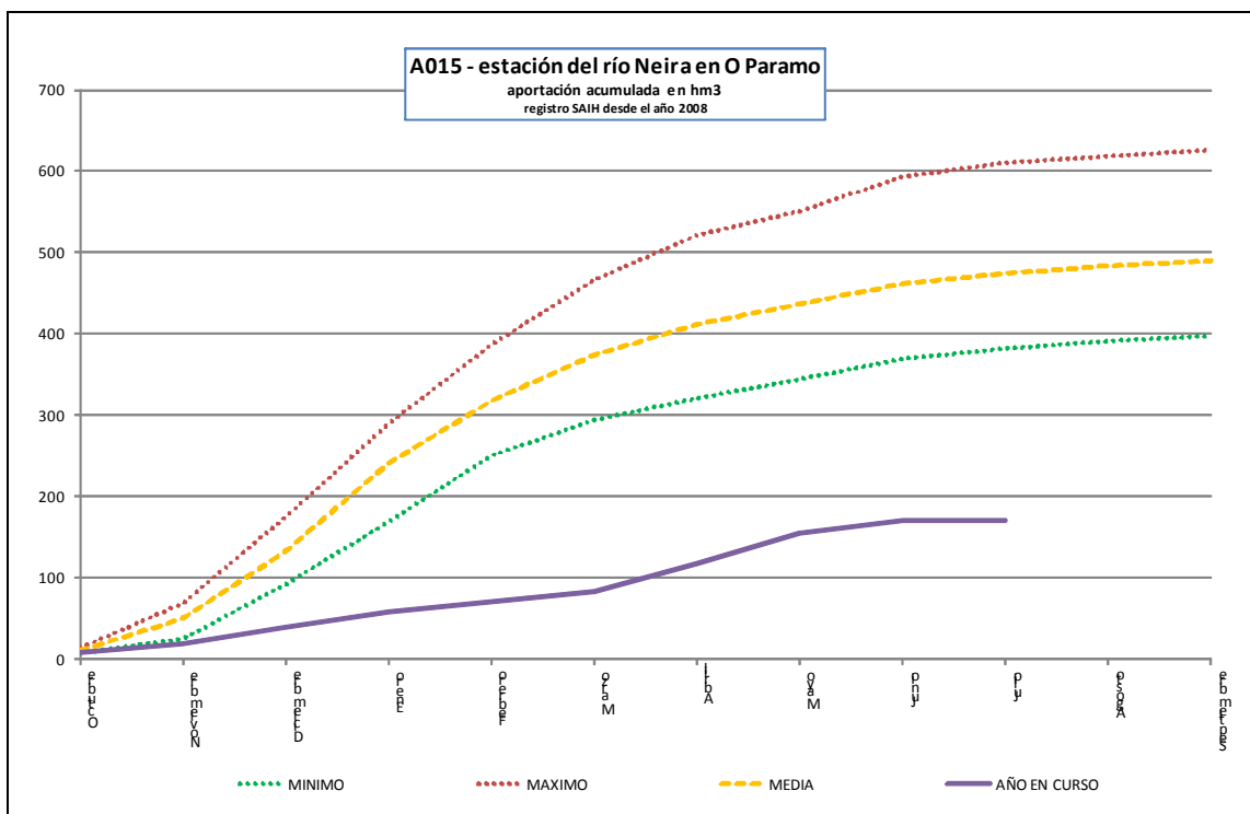
Estación de aforo A015 del río Neira en O Paramo
