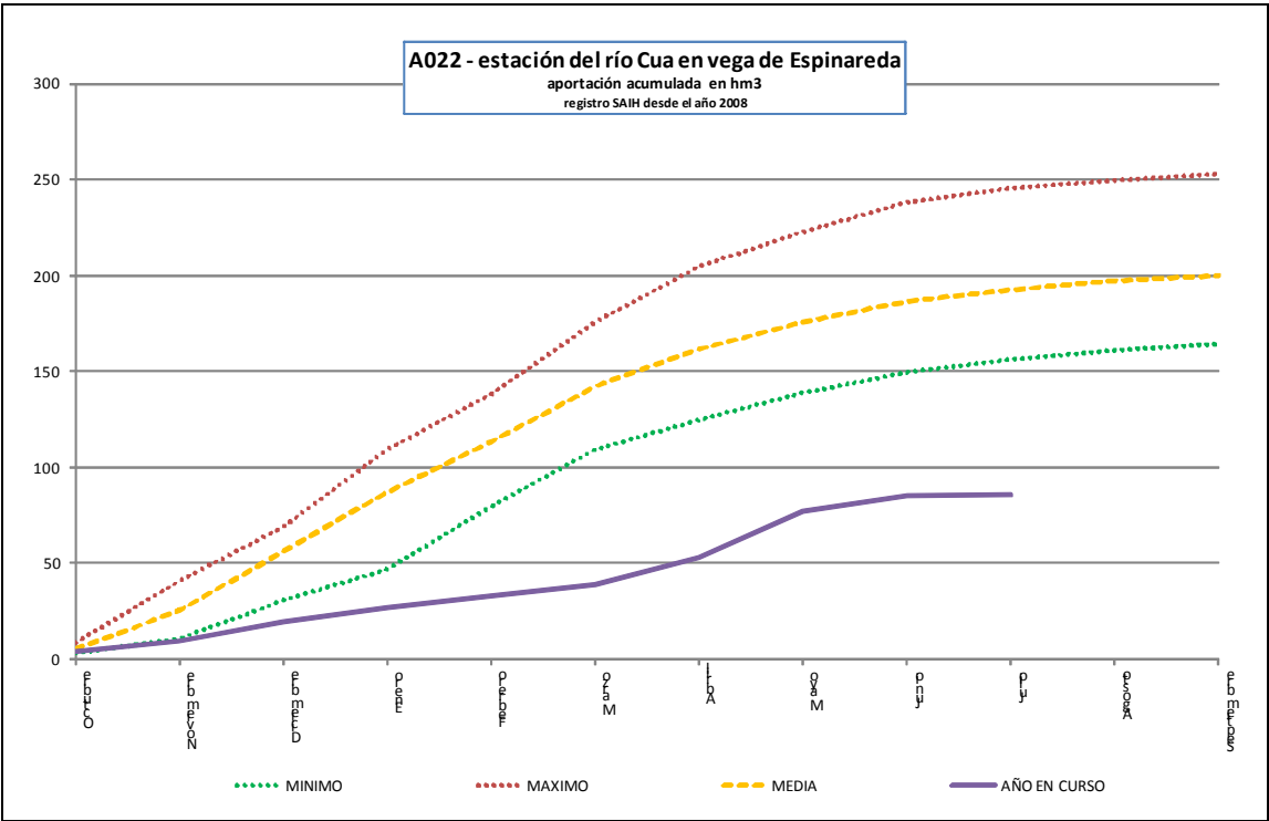
Estación de aforo A022 del río Cúa en Vega de Espinareda
