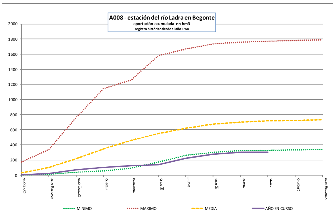
Estación de aforo A008 del río Ladra en Begonte
