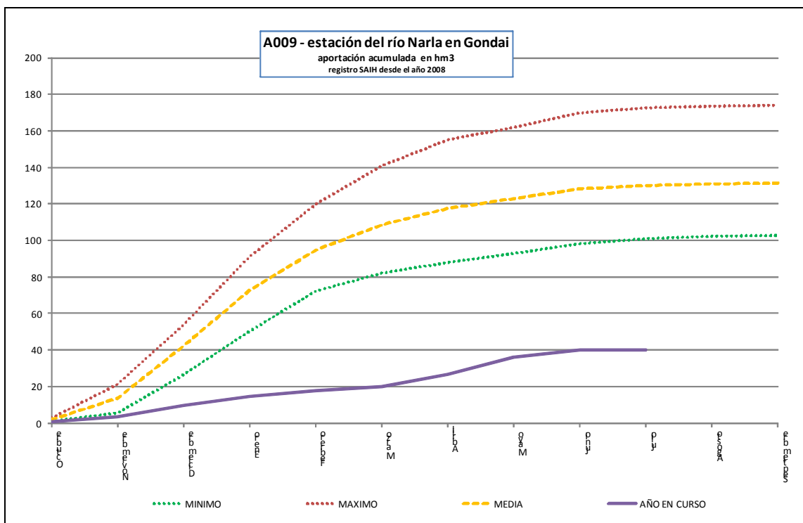
Estación de aforo A009 del río Narla en Gondai
