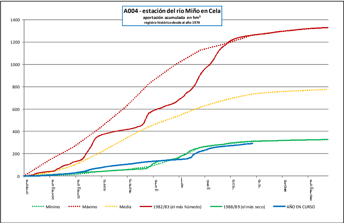
Estación de aforo A004 del río Miño en Cela
