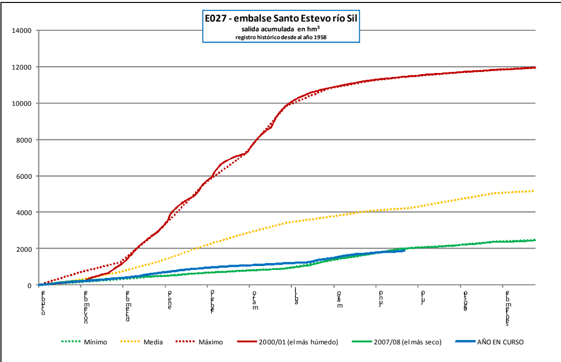
Embalse de Santo Estevo (Caudales de salida al río)
