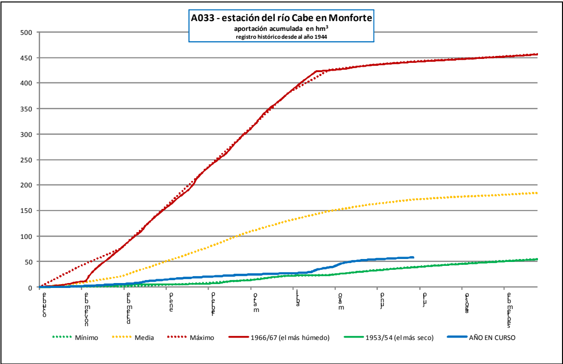
Estación de aforo A033 del río Cabe en Monforte
