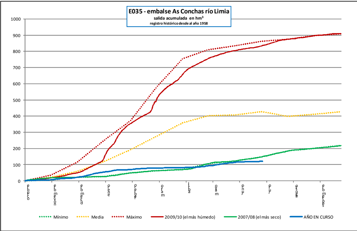
Embalse E035 del río Limia en As Conchas (Caudales de salida al río)
