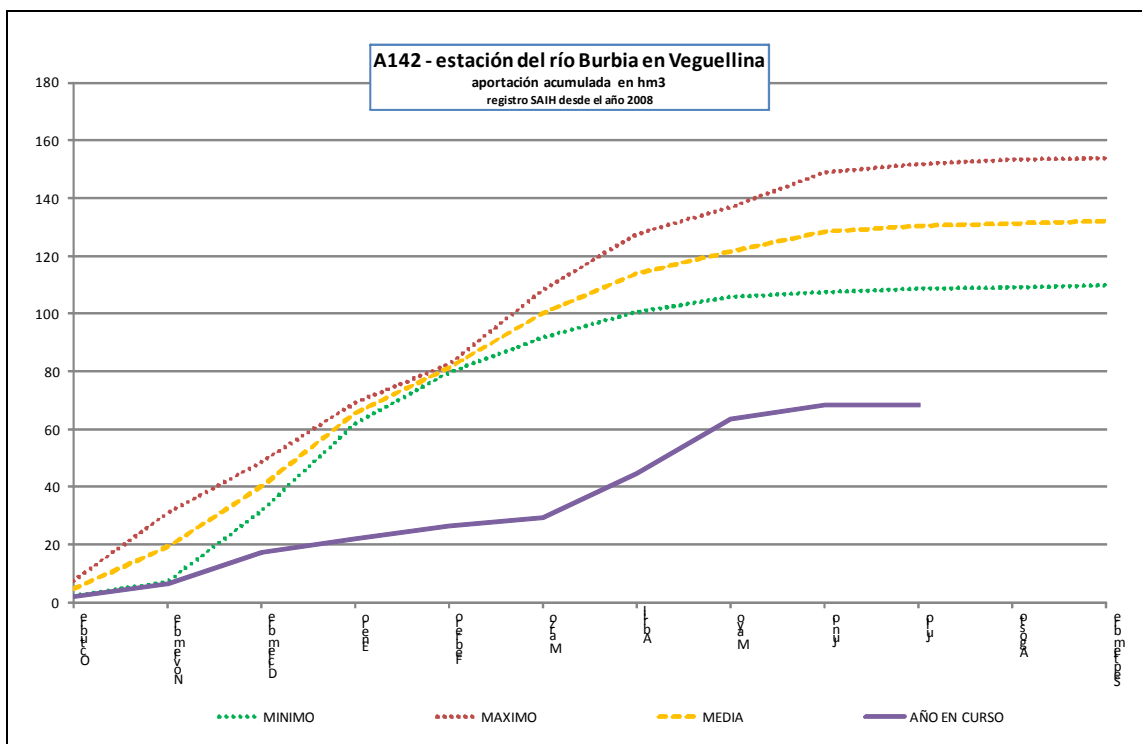
Estación de aforo A142 del río Burbia en Veguellina
