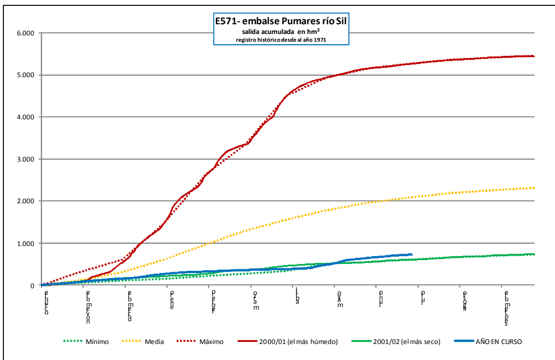
Embalse de Pumares (Caudales de salida al río)
