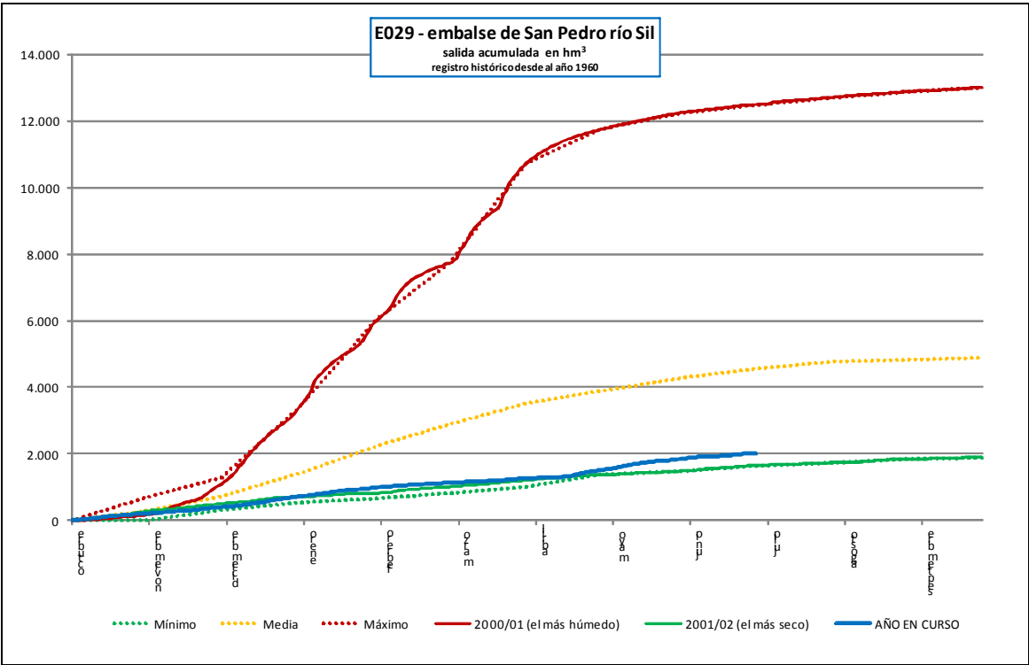
Embalse de San Pedro (Caudales de salida al río)
