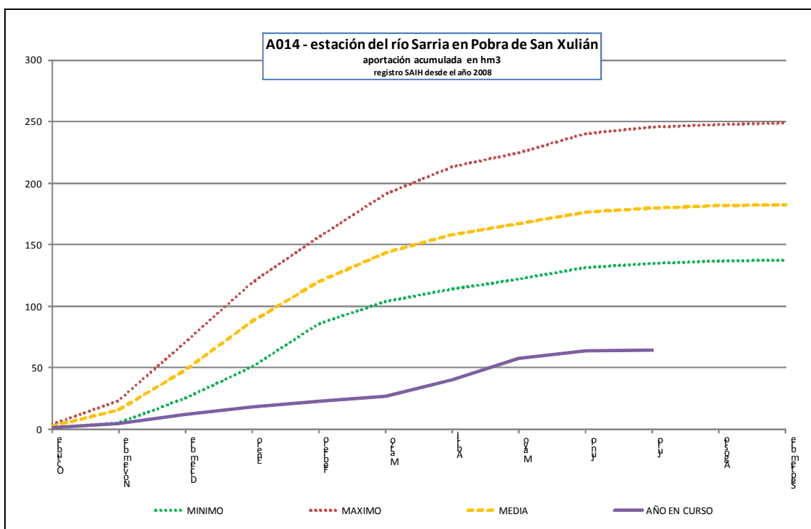
Estación de aforo A014 del río Sarria en Pobra de San Xulián
