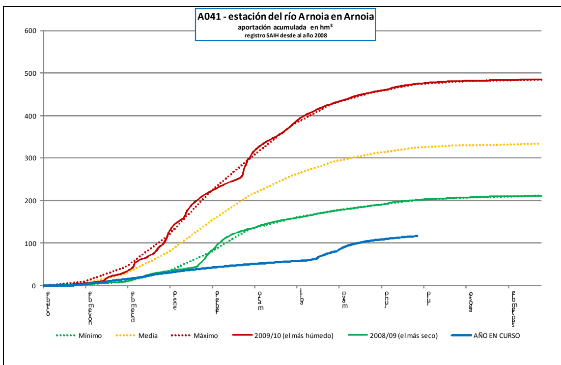
Estación de aforo A041 del río Arnoia en Arnoia
