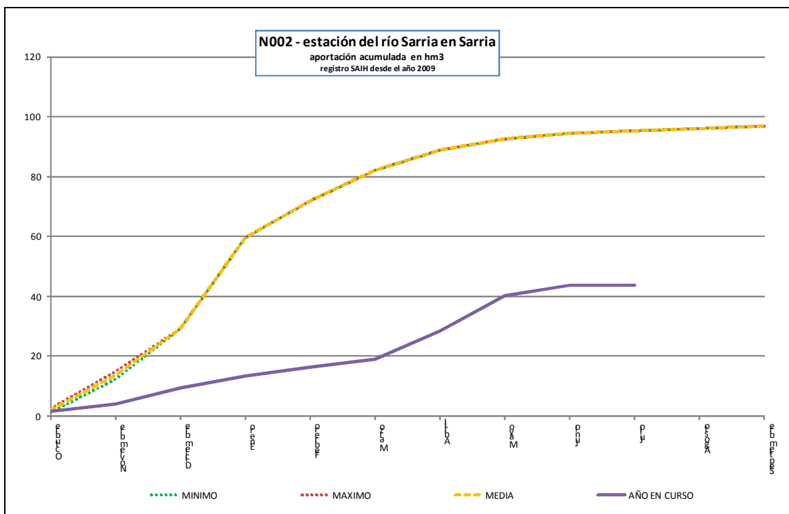
Estación de nivel N002 del río Sarria en Sarria (sólo se tiene completo el registro del año hidrológico 2010-2011)
