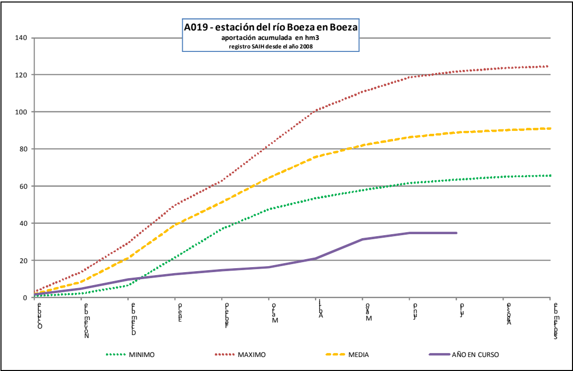
Estación de aforo A019 del río Boeza en Boeza
