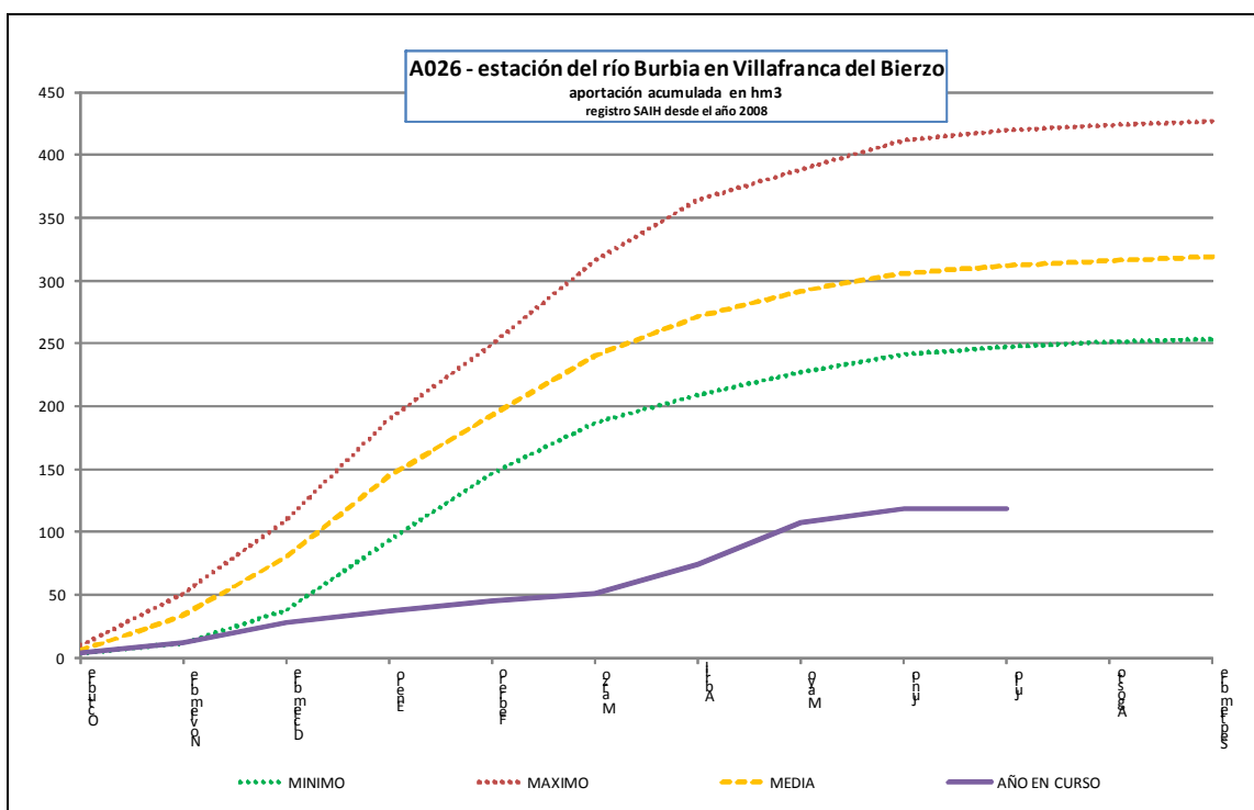
Estación de aforo A026 del río Burbia en Villafranca del Bierzo
