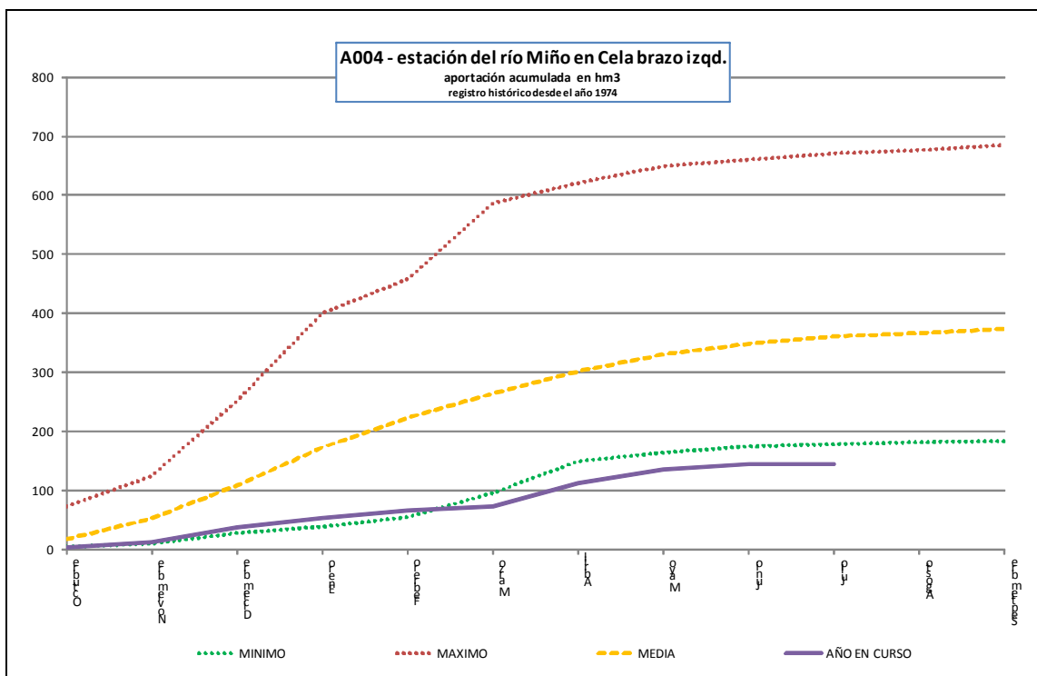
Estación de aforo A004 del río Miño en Ceta (brazo izquierdo)
