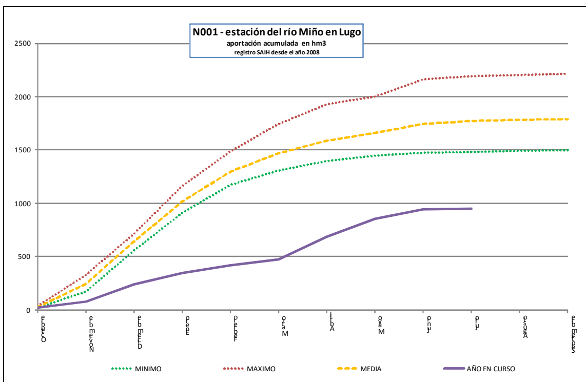
Estación de nivel N001 del río Miño en Lugo
